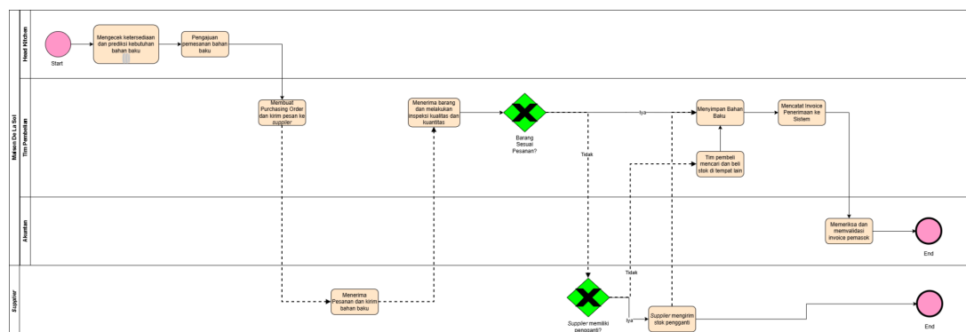
Gambar 2.4 BPMN Proses Pemesanan & Penerimaan Bahan Baku
